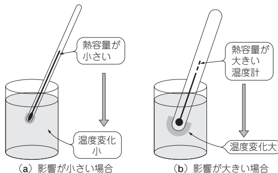
図8.1 温度計により測りたい温度が変わってしまう
