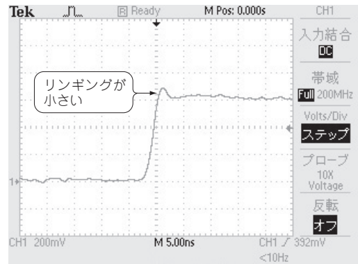
(b) 最短のグラウンド線
