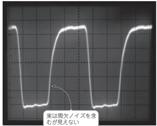
(a) アナログ・オシロスコープで測定した波形
