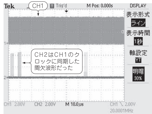
(b) (a) から時間レンジを長くするとCH2の波形が止まらない理由が見えた (10 μs/div)
